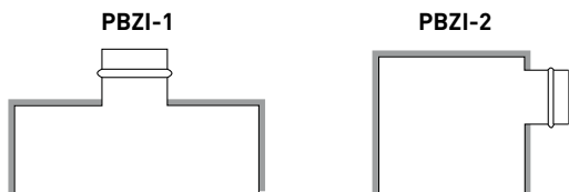
Plenum isolato esternamente spessore 6 mm Plenum externally insulated thickness 6 mm
