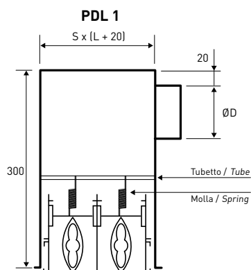
Fissaggio al plenum con molle CM Fixing to the plenum by springs CM
