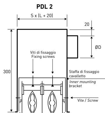
Fissaggio al plenum con staffe CVL cavalletti Fixing to the plenum by inner mounting brackets CVL
