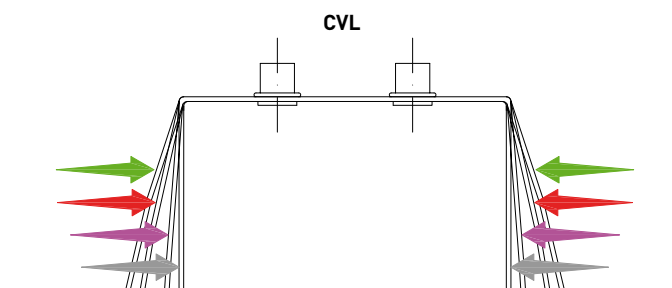
Modifica configurazione CVL da PDL 3 a PDL 2 con pressione delle dita Configuration change CVL to PDL 3 to PDL 2 with finger pressure
